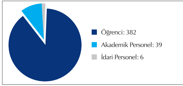
Şekil 2: Okuyucu İstatistiği
